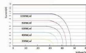
LNSF-335P/I-V
